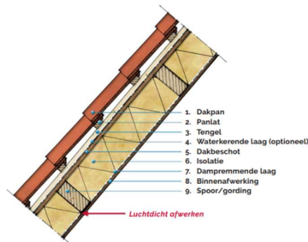
Isolatie en afwerking tussen de balken
