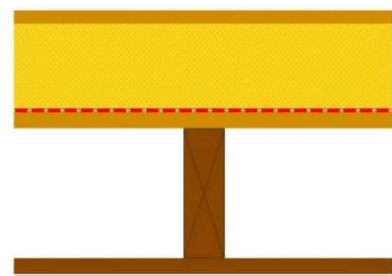
Dampdichte isolatie bovenop vloer
