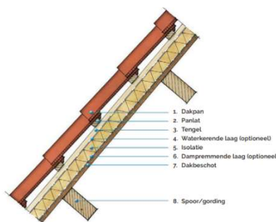
Harde isolatie op het dakbeschoot
