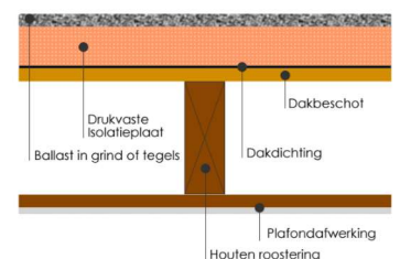
Omgekeerde dakisolatie
