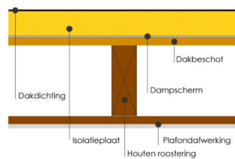
Warm dakisolatie
