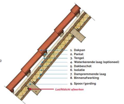
Isolatie tussen en afwerking over de balken
